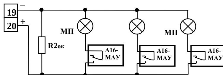
Рис.4. Схема подключения модулей пожаротушения ("МП") с контролем исправности цепи каждого модуля. R_{2ок} = 10 \text{ кОм} ( 0,25\text{Вт} , \pm 5\% ). При количестве модулей А16-МАУ более 4-х резистор R_{2ок} допускается не устанавливать.
