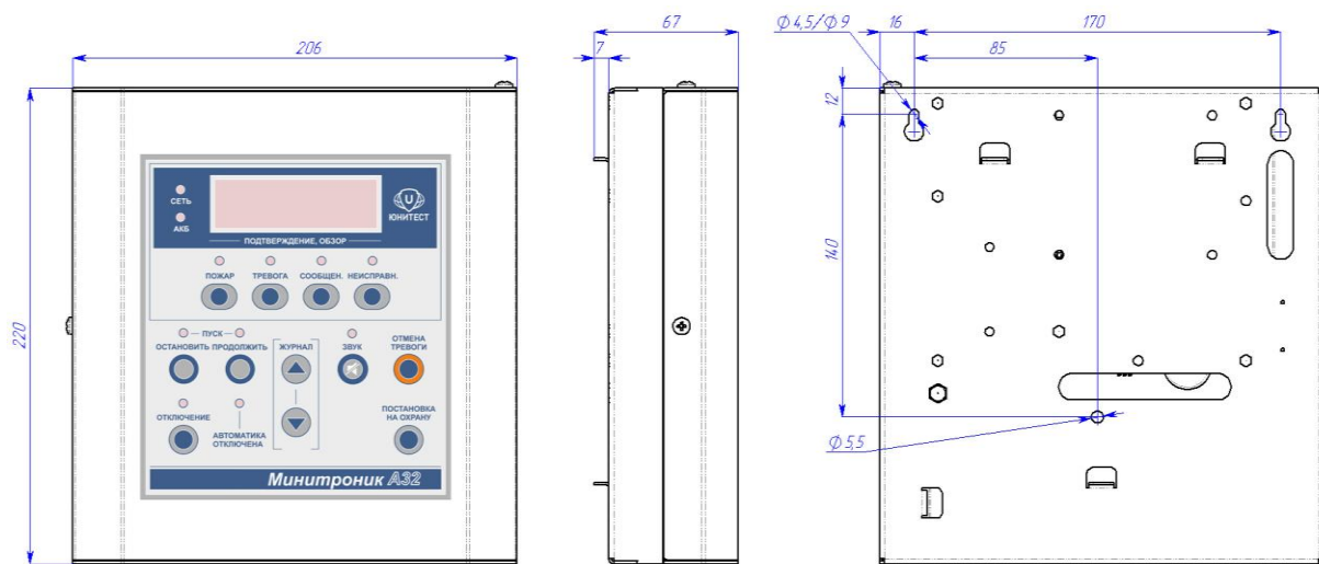
Рис.2. Габаритный чертеж и установочные размеры АПКП.
