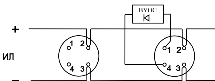
Рис.2. Схемы включения извещателя в адресную линию «Минитроник».
